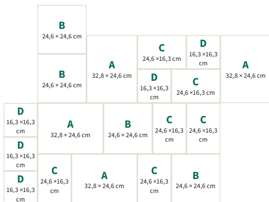
Wilder Verband 2
