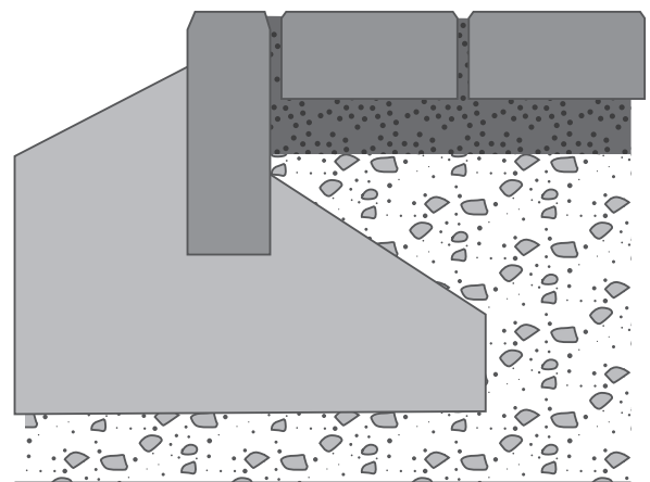
Randeinfassung
