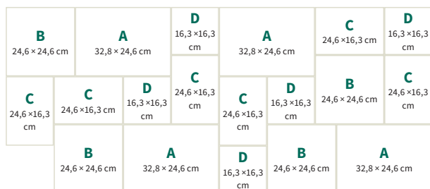
Wilder Verband 3
