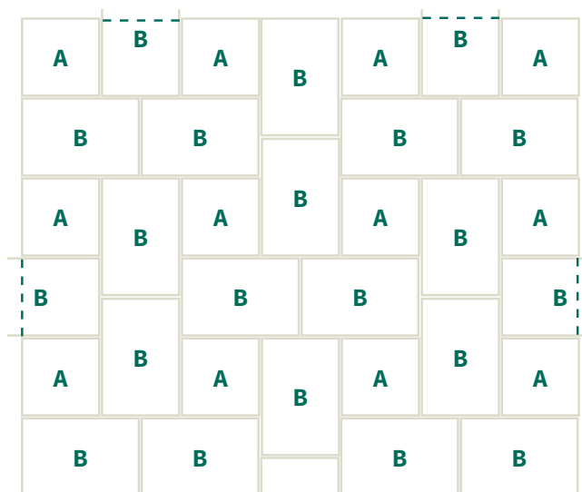
Kreuzverband
