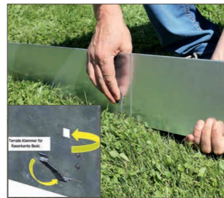
Schritt 1: Zwei Rasenkanten zusammenstecken.
