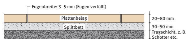
Plattenverlegung in ungebundenem Bettungsmaterial
