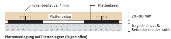
Plattenverlegung auf Plattenlagern (Fugen offen)
