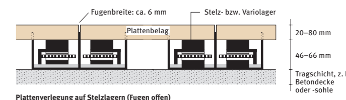
Plattenverlegung auf Stelzlagern (Fugen offen)
